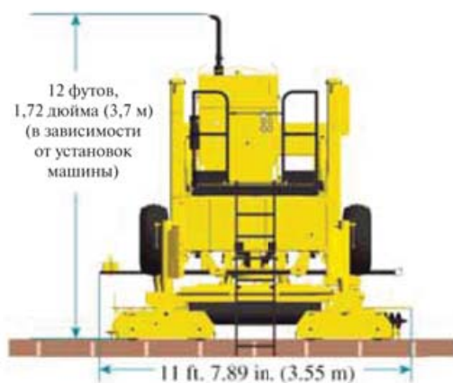
Формовой финишер С-650-Е, оборудованный катками
