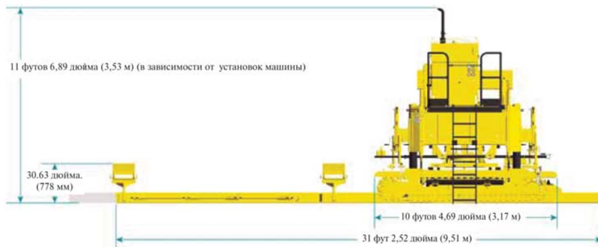
Финишер со скользящей опалубкой С-650-Е, оборудованный траками
